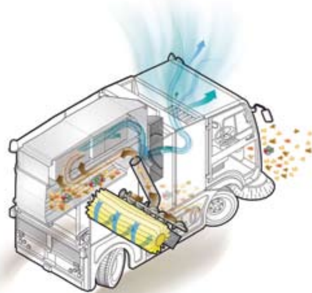
CS 140 Funktionsprinzip
